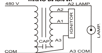
480 VOLT CONNECTION
