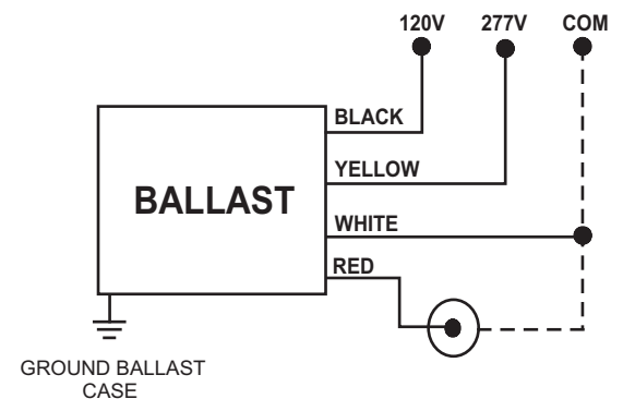
120/277 VOLT CONNECTION
